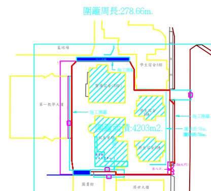
圍籬位置圖
