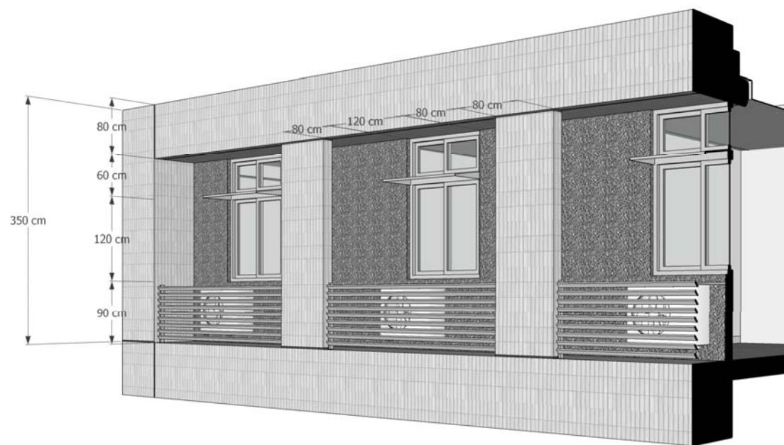
外牆系統(南、北向) 學生四人房/校友會館雙人房
