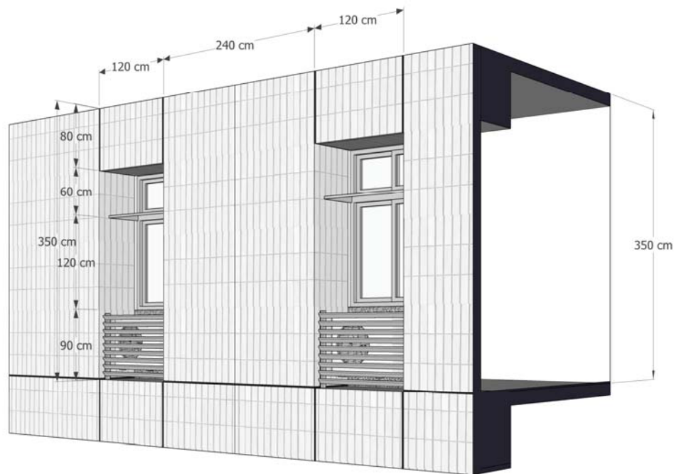
外牆系統(東、西向) 學生雙人房/校友會館一人房
